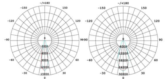
25X25 B/Angle BMP-5STAD25-800-1504-10D4 40X40 Angle BMP-5STAD40-800-1504-10D4
