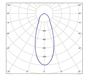
40x40 B/Angle BMP-FLMOD40-150-15057-10
