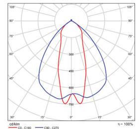
90x40 B/Angle BMP-HB2211-150-150V-10
