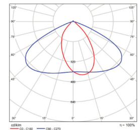
150x50 B/Angle BMP-HB2123-40-150V-10
