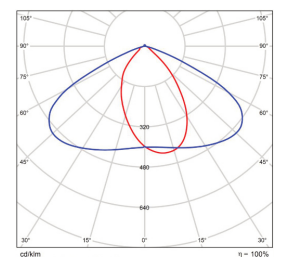
Tunnel Module BMP-SCAN2123-100-15057-10
