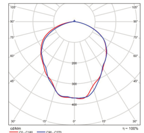
120x120 B/Angle BMP-SCAN150-150-15057-10D
