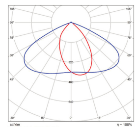
Tunnel Module BMP-SCAN2123-150-15057-10D
