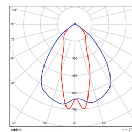
90x40 B/Angle BMP-SCAN2211-180-15057-10D
