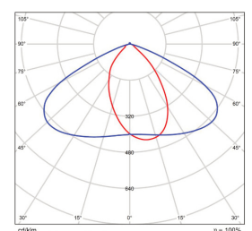
Tunnel Module BMP-SCAN2123-180-15057-10D
