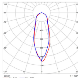
25 X 25 B/Angle BMP-STAD25-1000-150V-10D4
