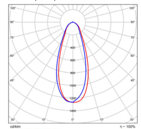
40x40 B/Angle BMP-STAD40-500-150V-10
