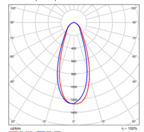
40x40 B/Angle BMP-STAD40-500-150V-10D4
