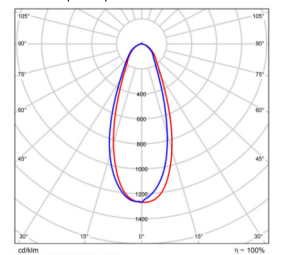
40x40 B/Angle BMP-STAD40-600-150V-10
