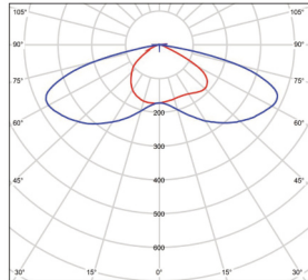
Type III BMP-STREET3-80-150V-10
