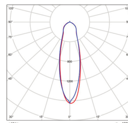
25x25 B/Angle BMP-FLMOD25-40-15057-10
